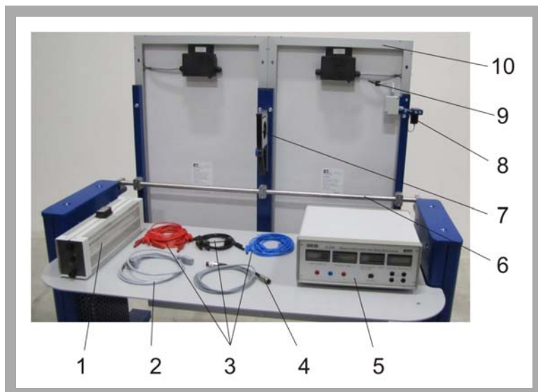
1 reóstato de cursor, 2 cable de red, 3 juego de cables para conexión en paralelo y en serie, 4 cable de medición, 5 unidad de medición, 6 eje basculante, 7 medidor de inclinación, 8 sensor de iluminancia, 9 sensor de temperatura, 10 módulos solares
