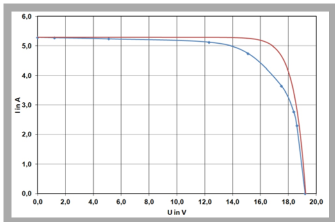
Curva característica de corriente y tensión de un módulo solar (temp. del módulo 55°C): medida (azul) teóricamente según el modelo de un diodo (rojo)
