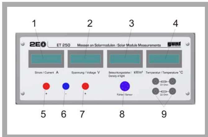
Indicadores: 1 corriente, 2 tensión, 3 iluminancia, 4 temperatura; Conexiones de medición: 5 corriente, 6 masa, 7 tensión, 8 iluminancia y temperatura, 9 resistores de potencia
