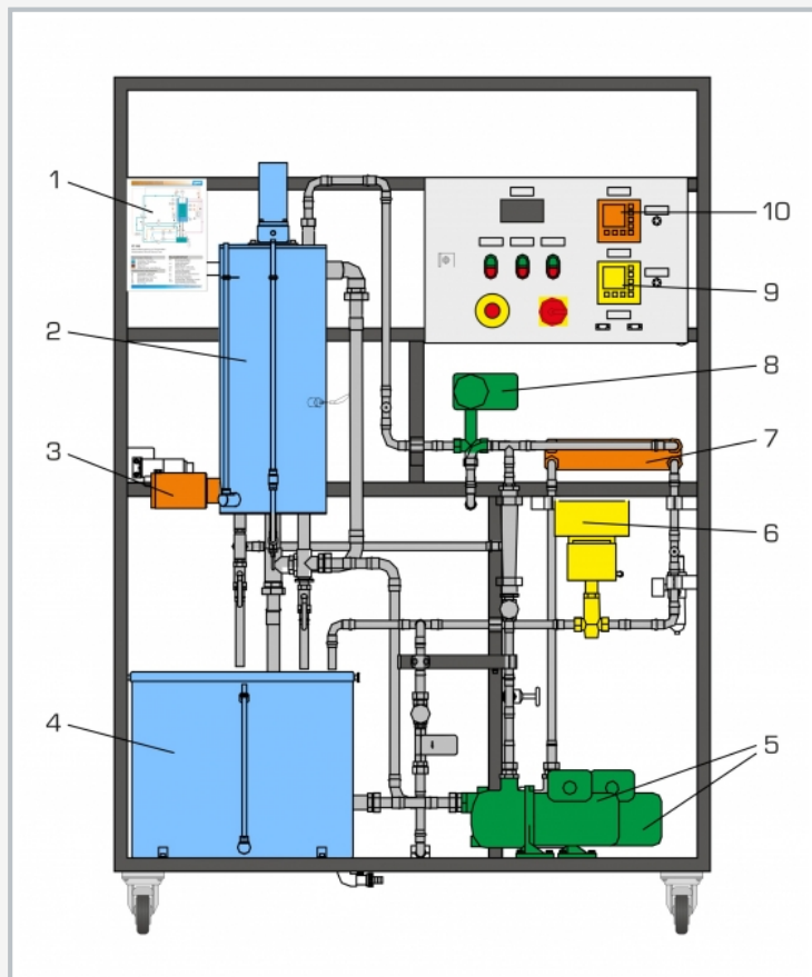
1 esquema de proceso, 2 depósito de agitación, 3 dispositivo de calefacción, 4 depósito colector, 5 bombas, 6 válvula de control de nivel, 7 cambiador de calor, 8 válvula de tres vías motorizada, 9 regulador de nivel, 10 regulador de temperatura
