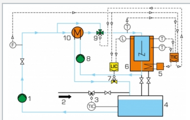
1 bomba del circuito principal, 2 agua refrigerante externa, 3 regulación de temperatura del depósito colector, 4 depósito colector, 5 dispositivo de calefacción, 6 depósito de agitación, 7 válvula de control de nivel, 8 bomba de precalentamiento, 9 válvula de tres vías motorizada, 10 cambiador de calor; F caudal, T temperatura, L nivel, LIC regulador (nivel), TIC regulador (temperatura)
