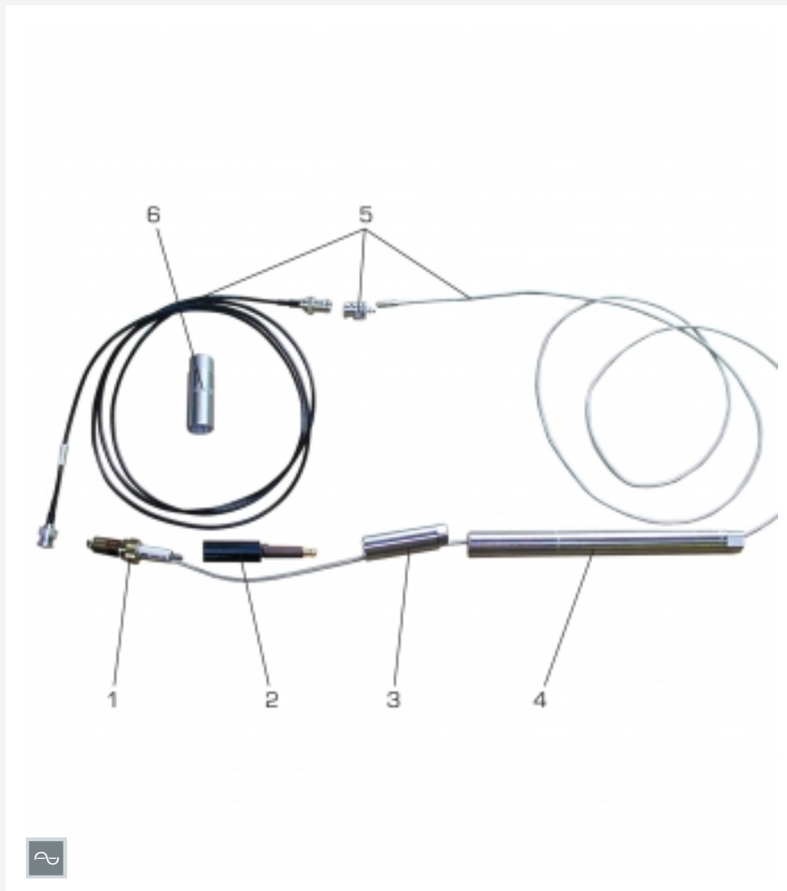
Die Abbildung zeigt einen ähnlichen Druckaufnehmer: 1 Zündkerze mit Druckaufnehmer, 2 Adapter, 3 Spezialsteckschlüssel, 4 Montagehilfe, 5 Anschlusskabel, 6 Steckschlüssel
