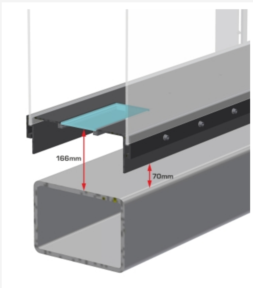
Einbaumaße für Lichtquelle oder Kamera unterhalb der Versuchsstrecke für ein kundeneigenes PIV-System
