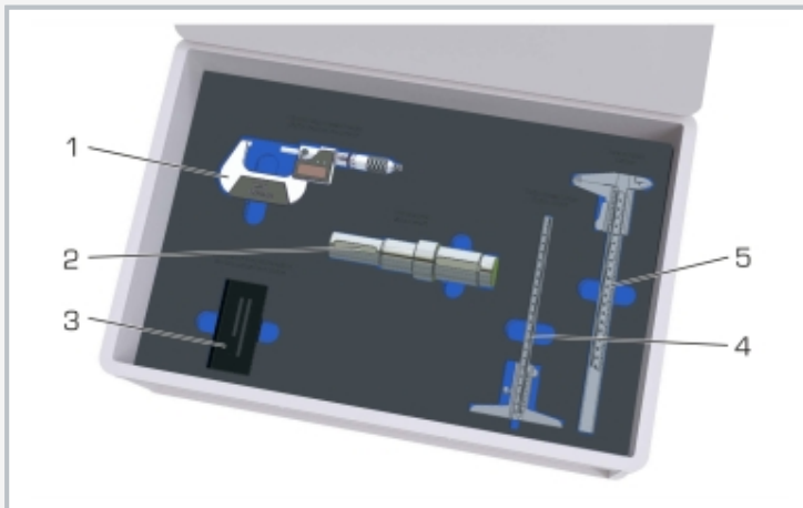
1 digitale Bügelmessschraube, 2 Prüfobjekt (Abtriebswelle), 3 Oberflächen-Vergleichsplatten, 4 Tiefenmessschieber, 5 Messschieber
