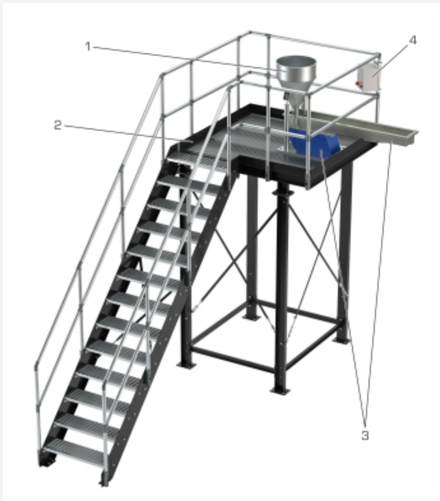
1 Trichter, 2 Bühne, 3 Feeder mit Schwingförderrinne, 4 Anschlussbox
