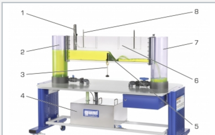
1 vanne plane, 2 alimentation en eau, 3 ajustage en hauteur du seuil, 4 réservoir de stockage, 5 déversoir à crête arrondie positionné dans le canal d'essai, 6 limite supérieure, 7 évacuation d'eau avec déversoir à paroi mince au niveau de la sortie d'eau, 8 tube de mesure
