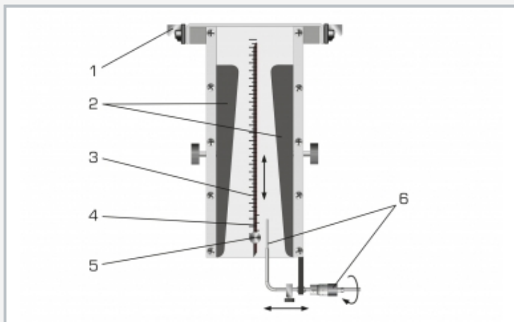
1 raccord rapide pour connexion sur HM 225, 2 corps latéraux démontables, 3 échelle graduée, 4 plaque avec différentes surfaces, 5 ajustage vertical de la plaque, 6 tube de Pitot avec vis micrométrique pour l'ajustage horizontal
