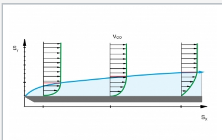
Répartition de la vitesse et épaisseur de la couche limite d'une plaque de surface plane, soumise à un écoulement incident longitudinal; écart S_y par rapport à la surface, écart S_x par rapport à l'arête avant, en vert: répartition de la vitesse, en bleu: épaisseur de la couche limite
