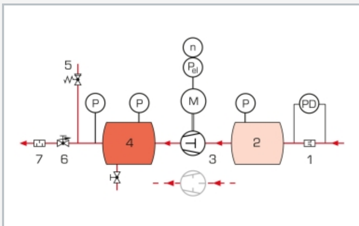
Essais (compresseur): 1 tube de Venturi (mesure du débit), 2 réservoir de stabilisation, 3 compresseur avec moteur d'entraînement, 4 réservoir sous pression, 5 soupape de sécurité, 6 soupape (ajustage du débit), 7 silencieux; P pression, PD pression différentielle, P_{ej} puissance, n vitesse de rotation
