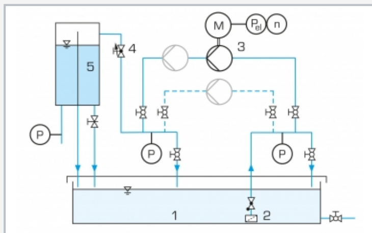
Essais (pompes centrifuges): 1 réservoir de stockage, 2 collecteur d'impuretés, 3 pompe avec moteur d'entraînement, 4 soupape (ajustage du débit), 5 réservoir de mesure; P pression, n vitesse de rotation, P_{el} puissance
