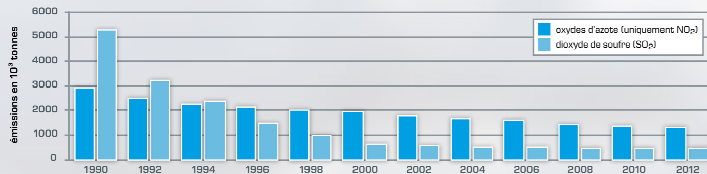
Émissions de dioxyde de soufre (SO 2 ) et d'oxydes d'azote (uniquement NO 2 ) en Allemagne Source: Umweltbundesamt (Ministère de l'environnement allemand), tableaux nationaux de tendances de l'étude allemande sur les émissions atmosphériques (version 2014)
