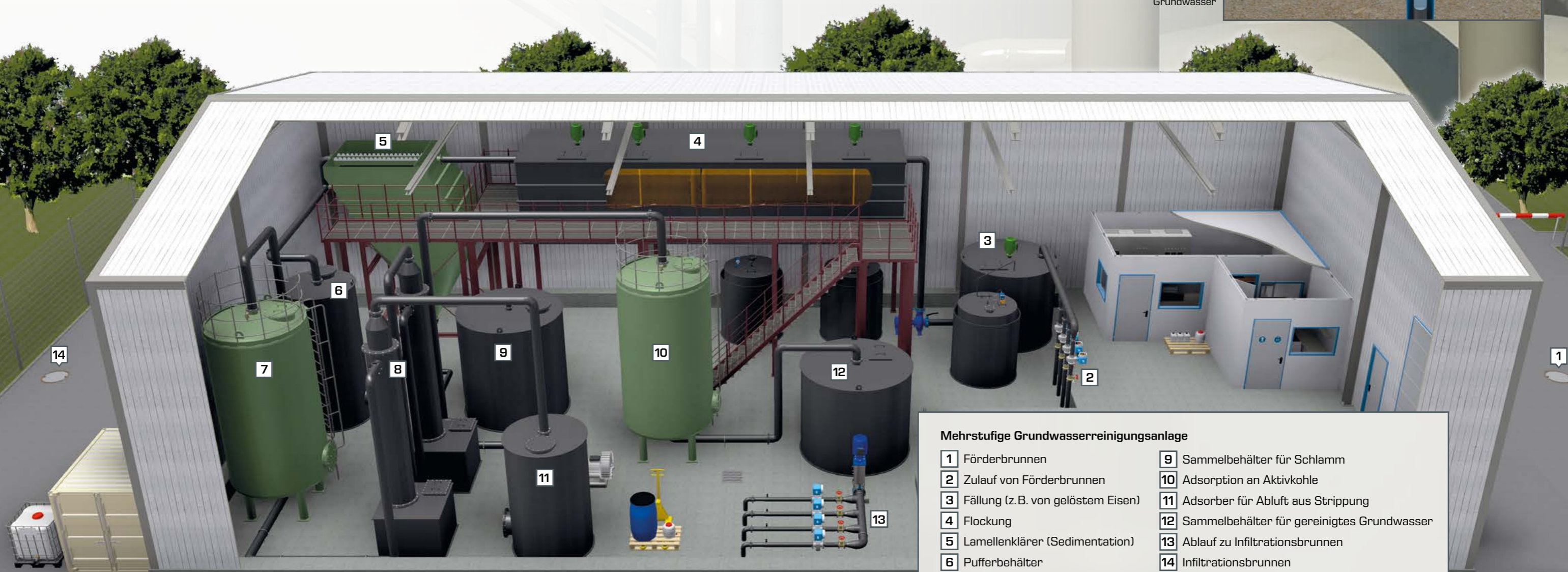
Förderbrunnen für kontaminiertes Grundwasser
