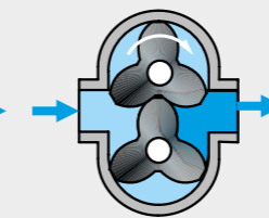
Pompe à piston tournant
