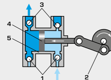
Pompe à piston
